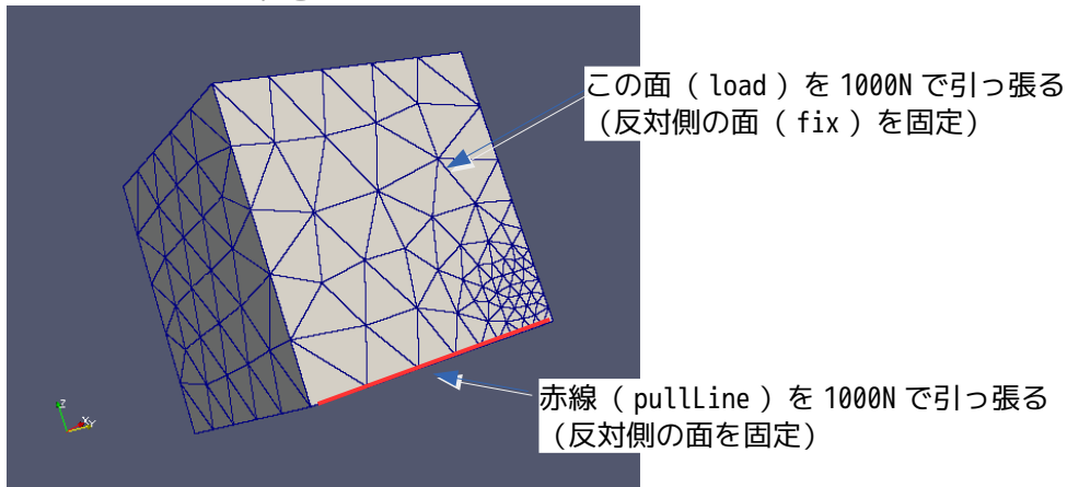
メッシュの状態
