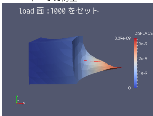
<四面体1次要素の場合> トータル荷重
