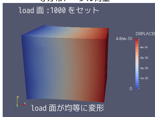
等分布トータル荷重
