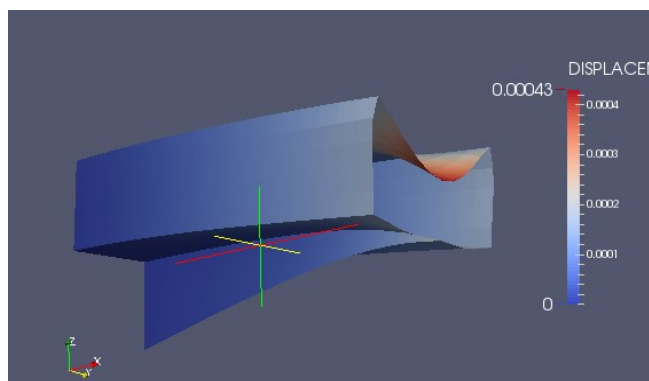
mises 応力
