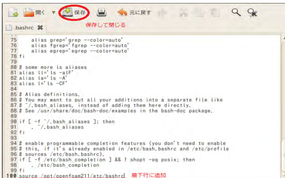
図 15 ./bashrc ファイル
